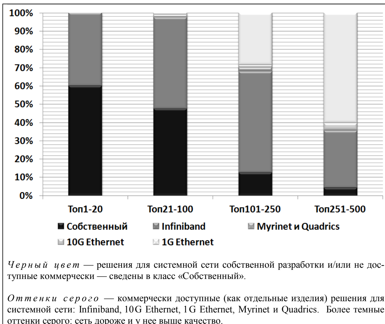
Рисунок 2. Доли использования различных технологий для системной сети в суперкомпьютерах различного уровня производительности (июньская редакция рейтинга Top500 2012 года)
