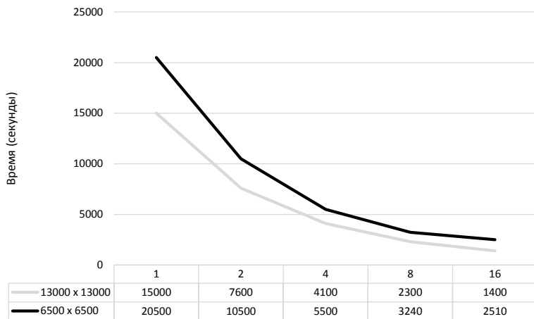
Рис. 4. График зависимости ускорения исполнения от количества узлов
