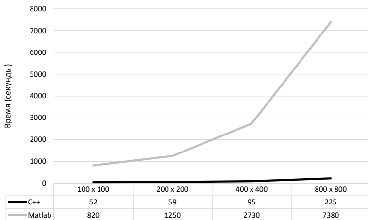
Рис. 2. Сравнение времени исполнения программы на разных языках
