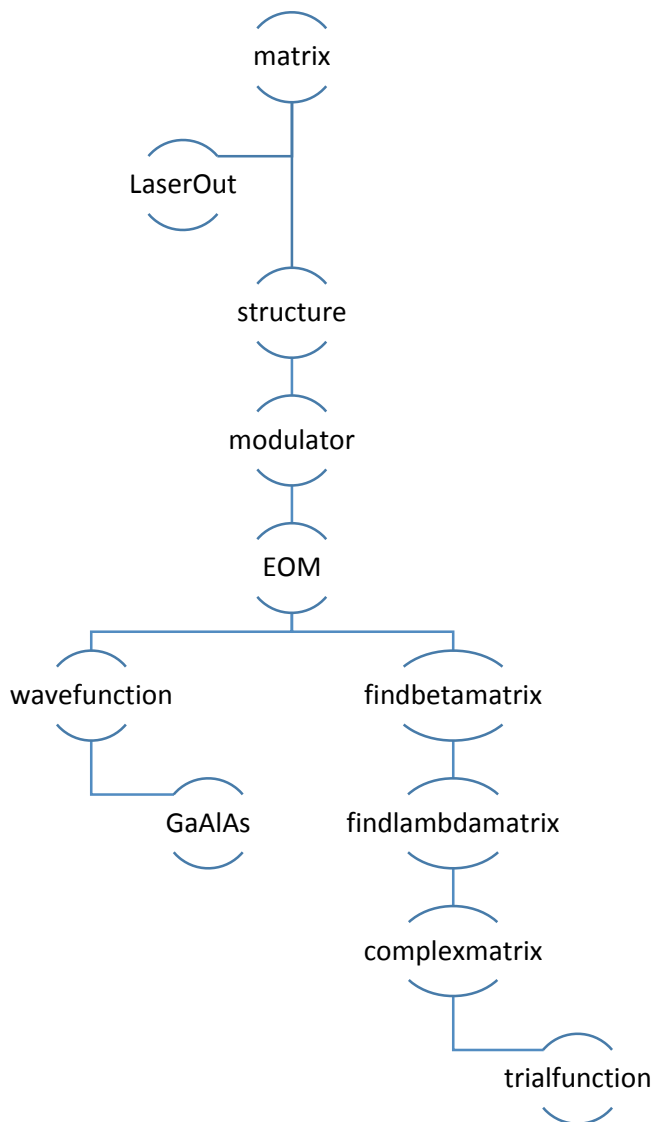
Рис. 1. Граф вызова функций в изначальной программе
