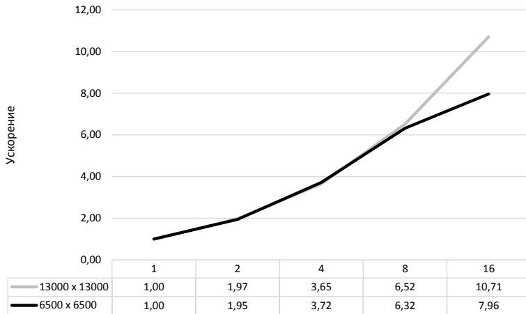
Рис. 3. График зависимости времени исполнения от количества узлов
